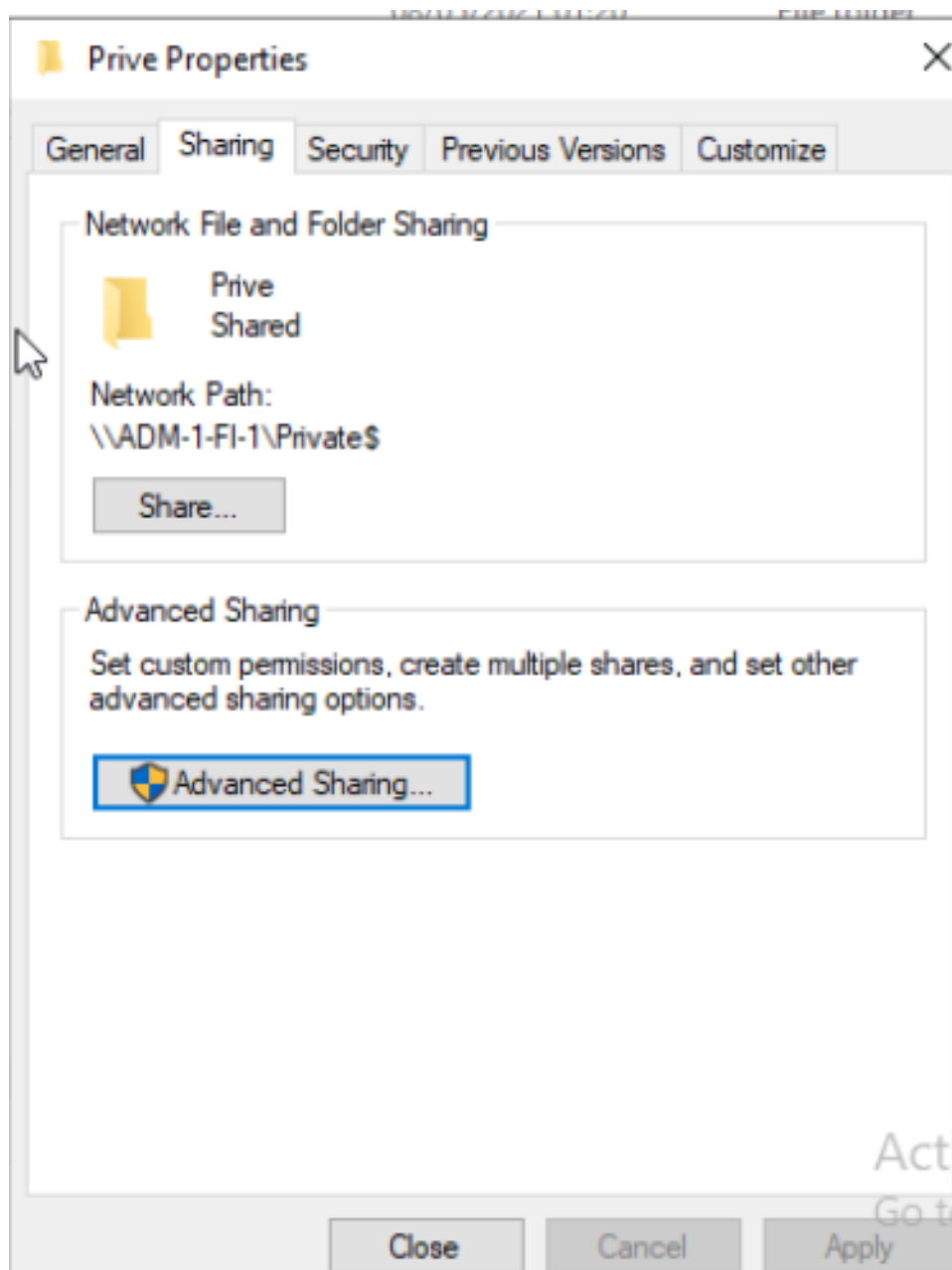
Partage du dossier Prive — nom masqué avec $ — permissions de modification
