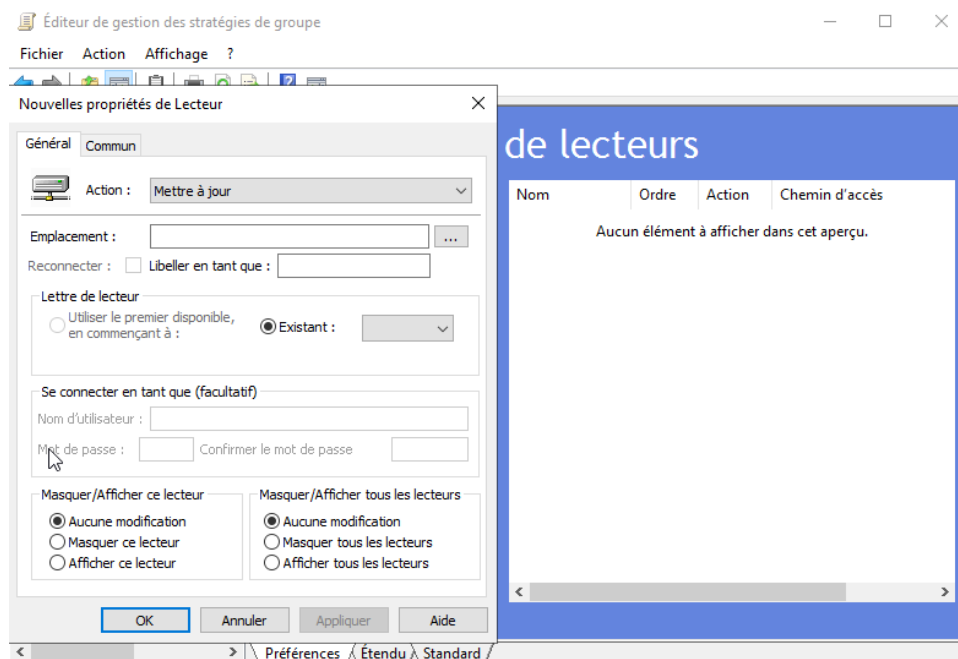
Paramétrage du lecteur réseau — chemin UNC du dossier partagé
