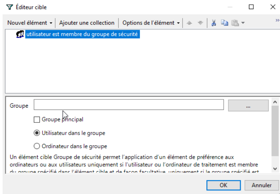
Ciblage du mappage lecteur sur un groupe de sécurité spécifique
