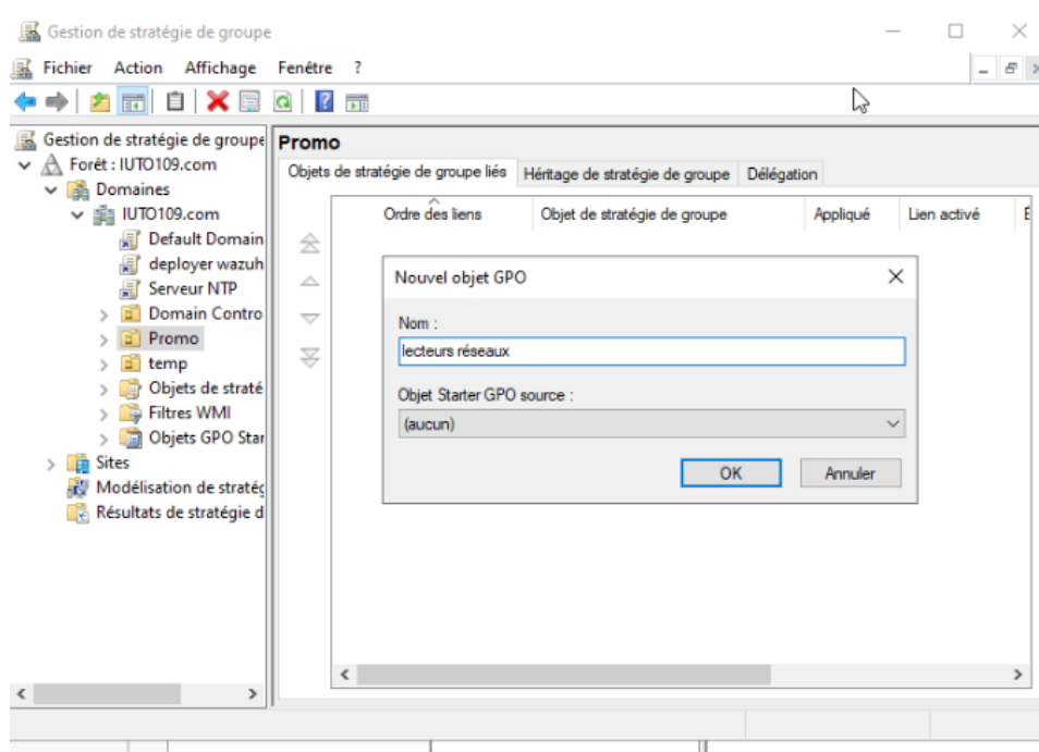
Création et liaison de l'objet GPO sur l'OU promo
