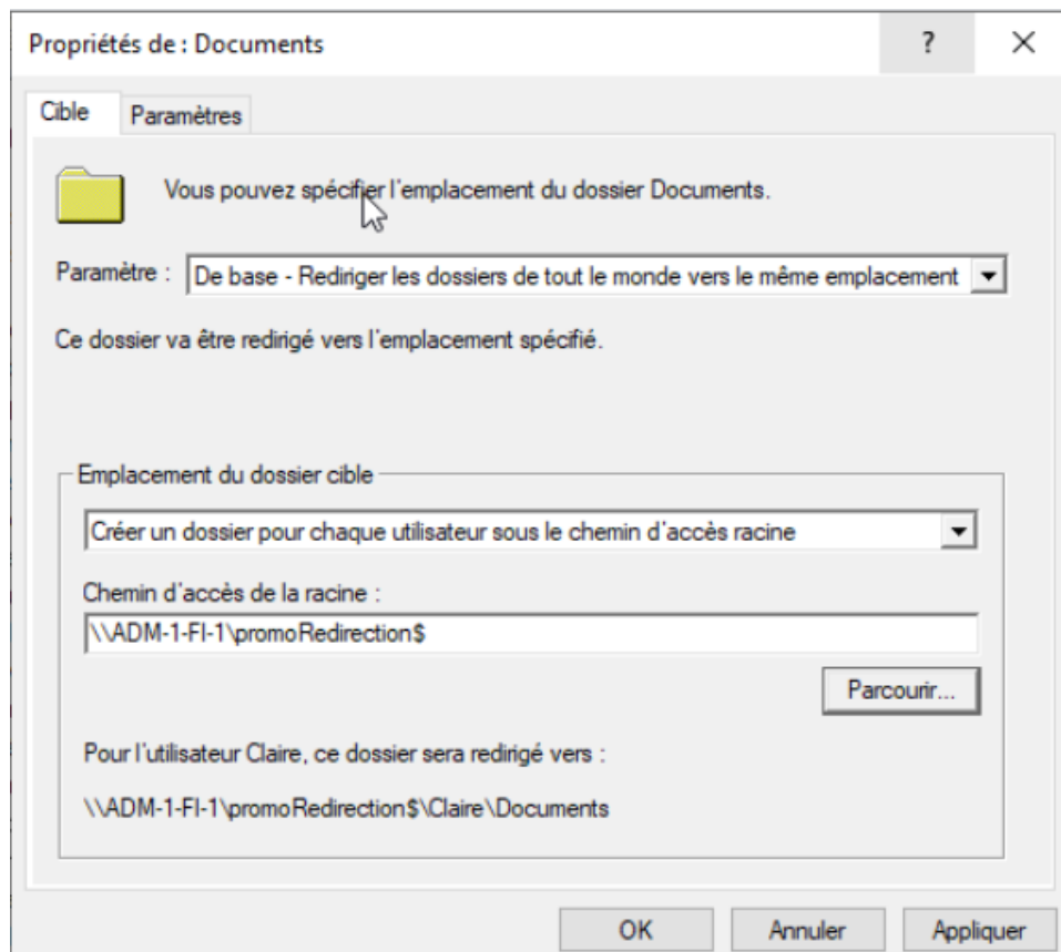
Configuration de la redirection du dossier Documents
